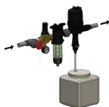
Installation en ligne
